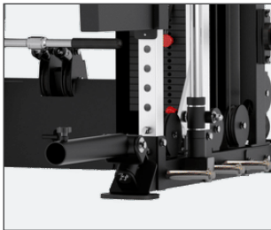
El rack de entrenamiento Smith es ajustable con 16 posiciones y Land Mine.
