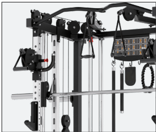
Con 30 posiciones ajustables, cada una separada por 5 cm. La posición más alta alcanza los 180 cm del suelo y la más alta los 33 cm, afiche con instructivo de ejercicios.
